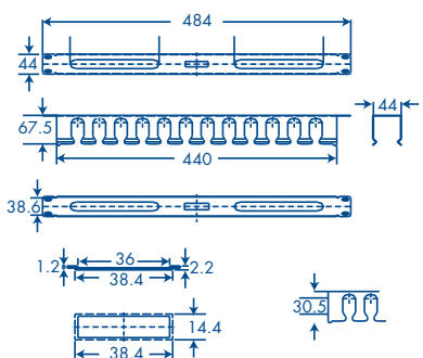
ORGANIZADOR DE CABLES 1U DE RACK CON TAPA METÁLICA ABATIBLE
