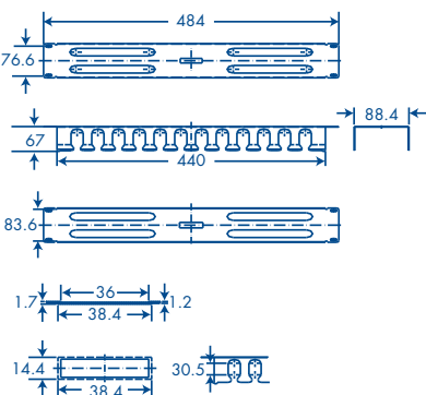
ORGANIZADOR DE CABLES 2U DE RACK CON TAPA METÁLICA ABATIBLE
