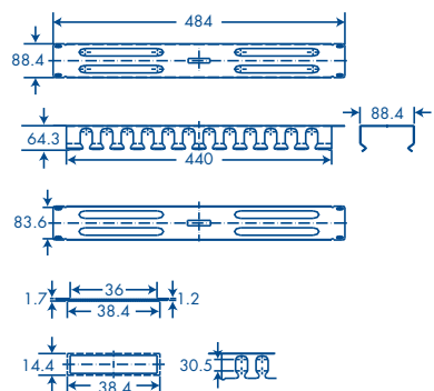
ORGANIZADOR DE CABLES 2U DE RACK CON TAPA DE PVC MOVIBLE
