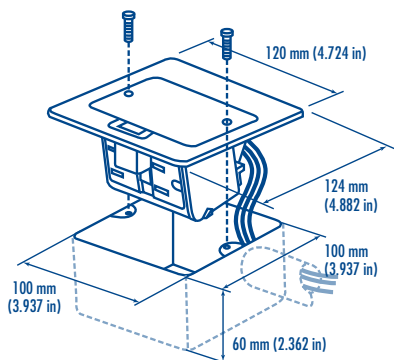
Mini caja de piso de contactos rectangular
