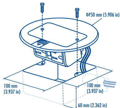
Mini caja de piso de contactos redonda
